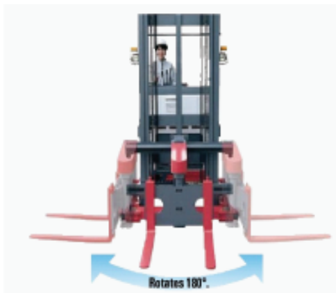
采用意大利ZAIPI AC控制器,全液压助力转向, 通过多路阀轻松控制旋转头左右180度旋转。
