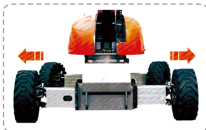
>> 伸展轮轴
